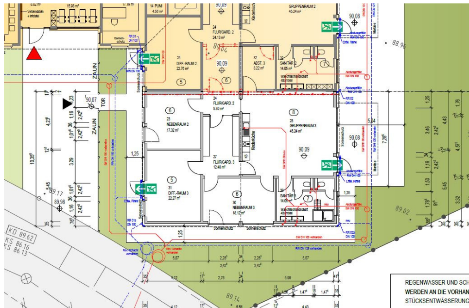
Grundriss Anbau 3. Gruppe KiTa Pustebblume
